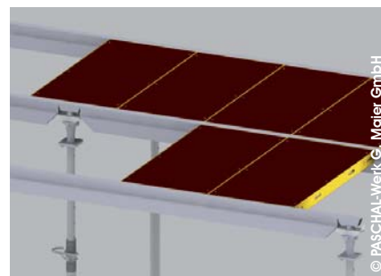
Вариант III Элементы монтируются в балки, при необходимости с опускающейся головкой.
