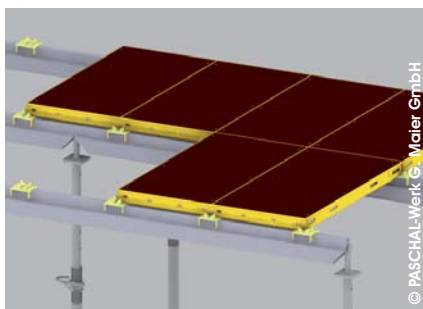
Вариант II Элементы монтируются на балки.
