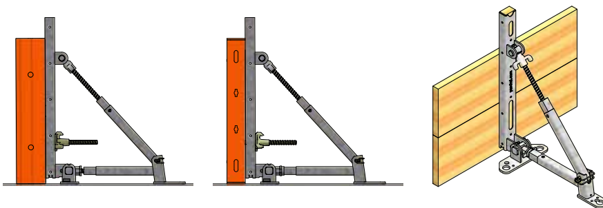
N189.001.0032 Gurthalterung 240 Klemmlänge 24cm N189.001.0031 Gurthalterung 100 Klemmlänge 10cm
