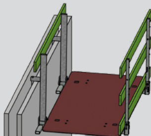
Betonierbühne mit Hohlwandadapter einhängen
