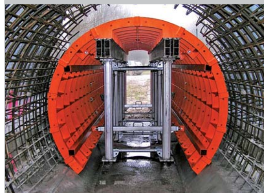
Передвижной стол для туннеля- Стягивающаяся опалубка с опорным каркасом ГАСС
