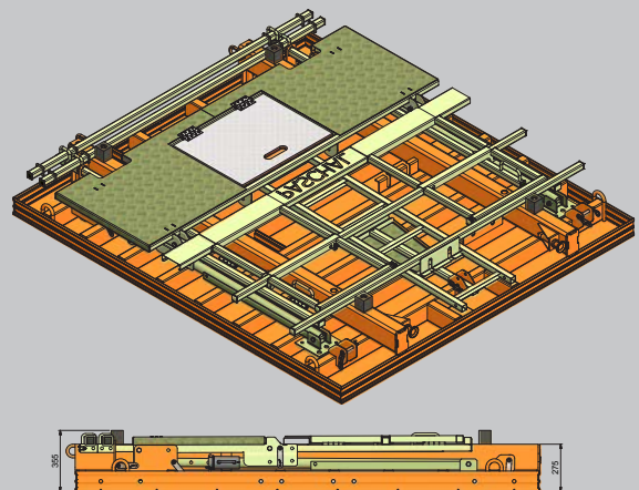
Die Elemente sind zusammengeklappt eine kompakte Einheit mit fest verbundener Sicherheitseinrichtung „Multip“.
