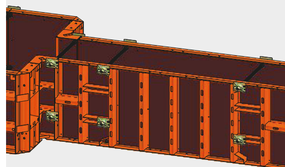
Das LOGO-Element 270 x 90 cm erlaubt eine Wahlmöglichkeit bei der Platzierung des Spannstabes.
